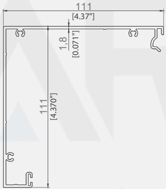
MOTOR KUTUSU PROFİLİ MOTOR BOX PROFILE
