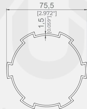
Motor Tüp Profili / Motor Tube Profile
