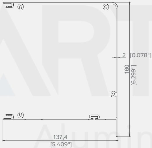
Motor Kutusu Profili / Motor Box Profile
